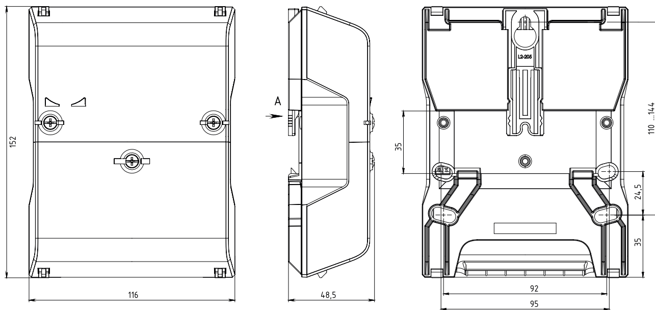
Рисунок 1 - Габаритные и установочные размеры
